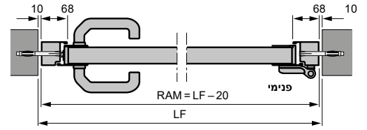
דלת צד עם מסגרת בלוק אלומיניום, פרופיל סוג 2 הרכבה בפתח
