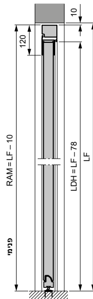
דלת צד עם מסגרת בלוק אלומיניום, פרופיל סוג 2 הרכבה בפתח
