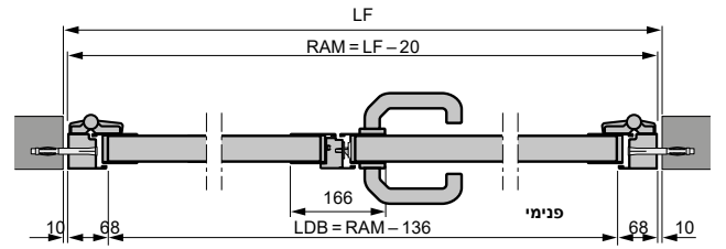
דלת צד בעלת 2 כנפיים עם מסגרת בלוק אלומיניום פרופיל סוג 2 הרכבה בפתח
