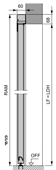
דלת צד עם מסגרת בלוק אלומיניום, פרופיל סוג 2 הרכבה מאחרי הפתח
