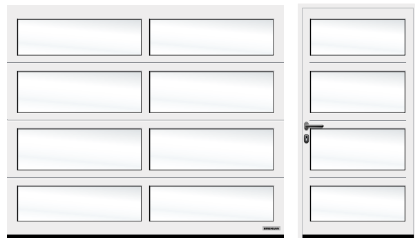
ART 42 צבע לבן מזוג, לבן RAL 9016
