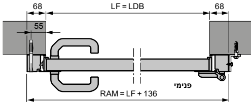
דלת צד עם מסגרת בלוק אלומיניום, פרופיל סוג 1 הרכבה מאחרי הפתח
