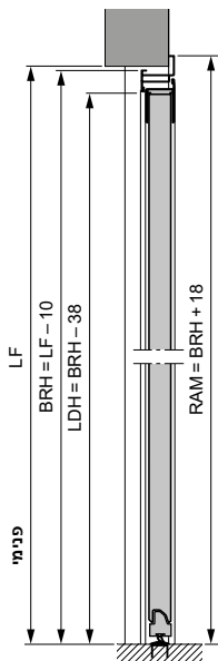
דלת צד עם מסגרת פינתית מאלומיניום, פרופיל סוג 2 מגרעת חיצונית
