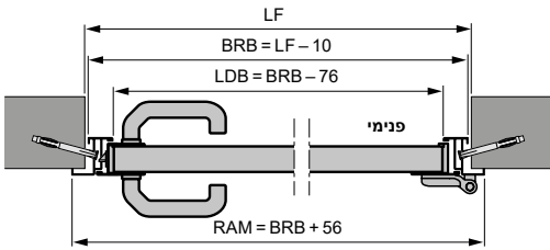
דלת צד עם מסגרת פינתית מאלומיניום פרופיל סוג 1 או 2 מגרעת פנימית
